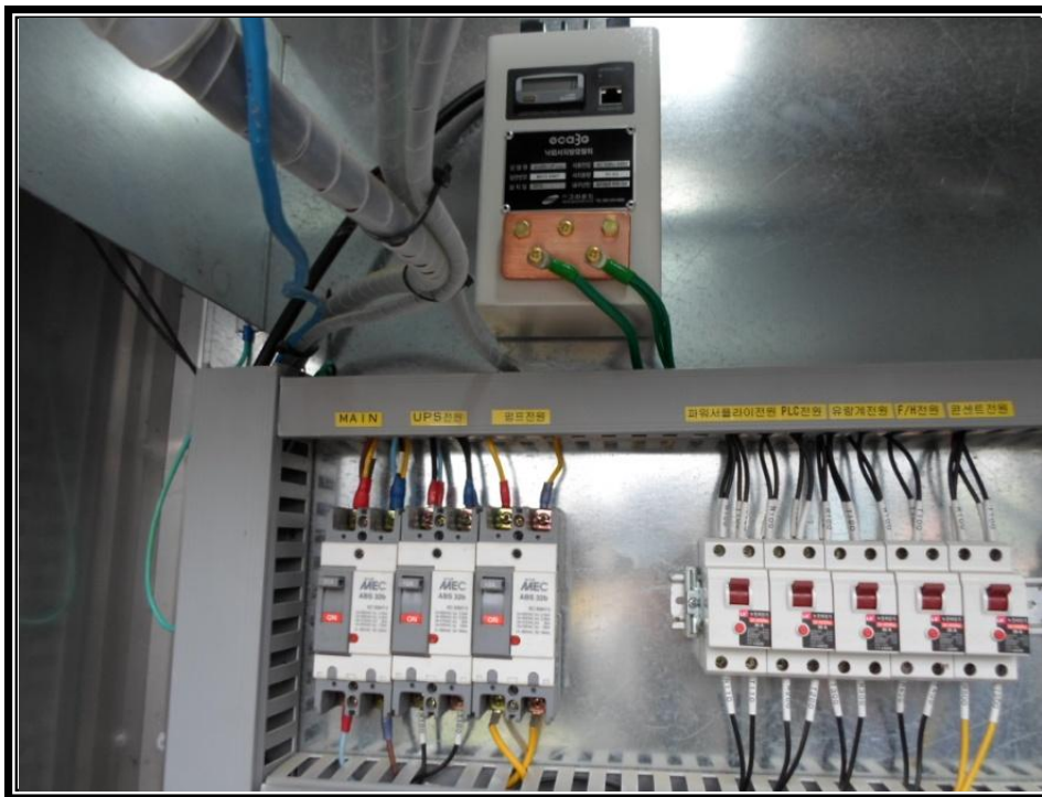
eca3G 설치 후 LP-1P(MS2)
