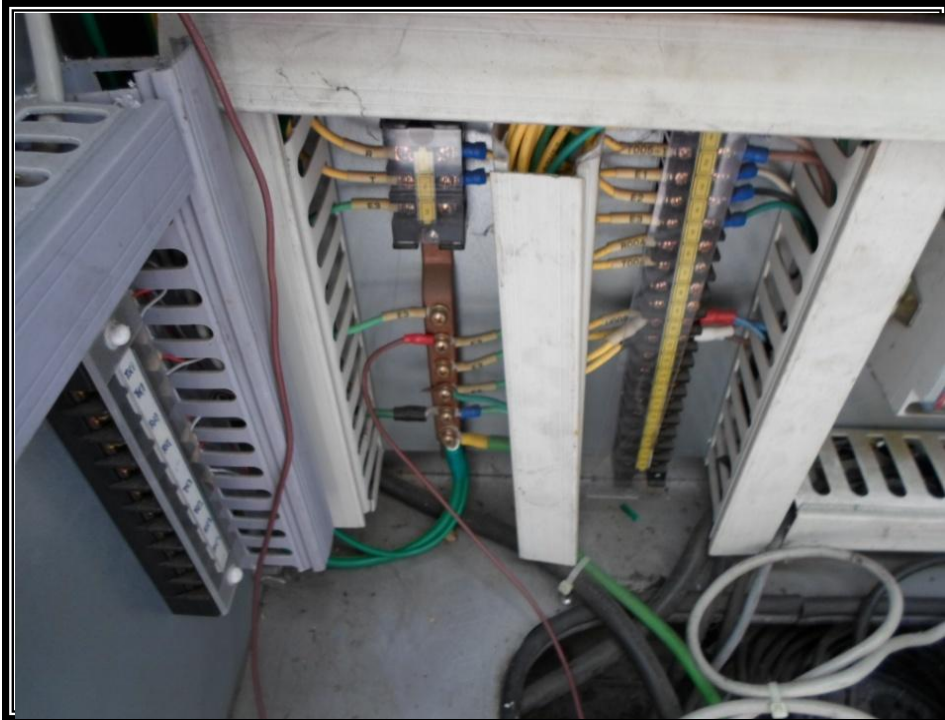
eca3G 설치 전 (MD1)
