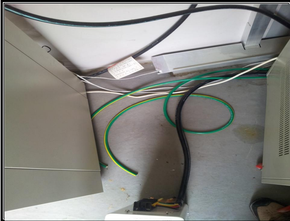
eca3G 설치 중(염소투입실)
