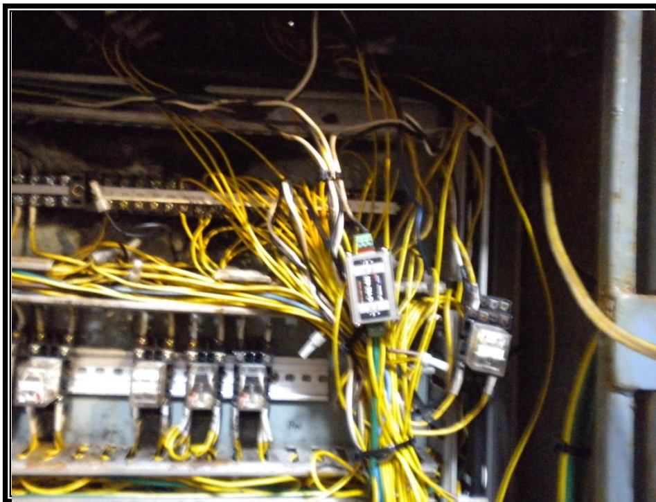
통신용 보호기설치
