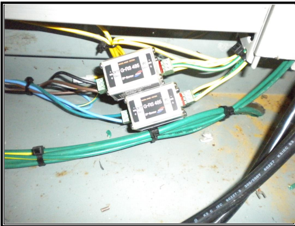
통신용 보호기설치
