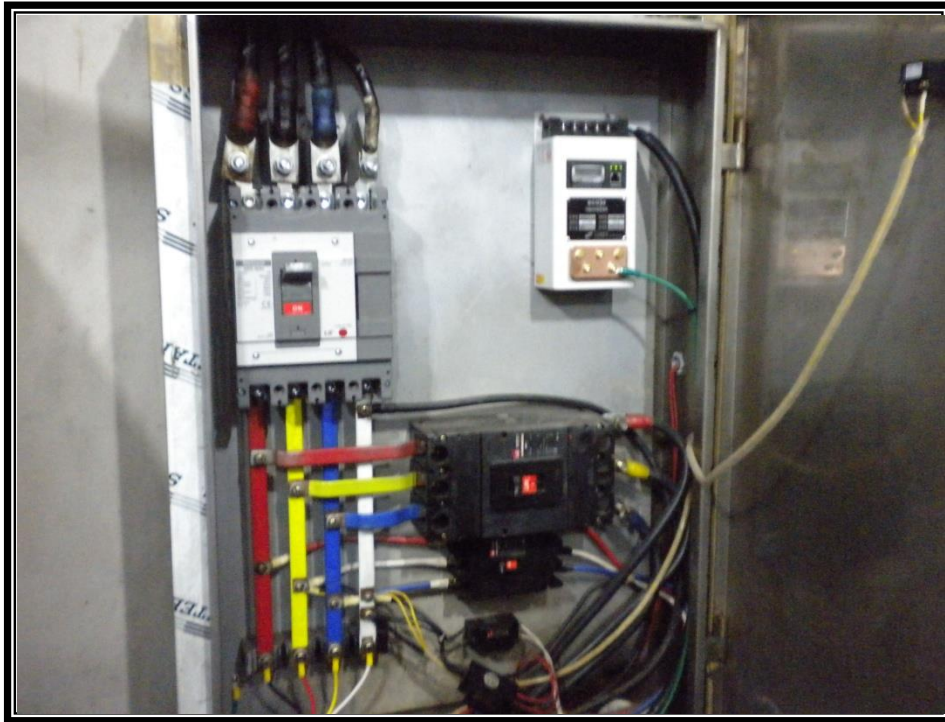
전원용LP설치-1
